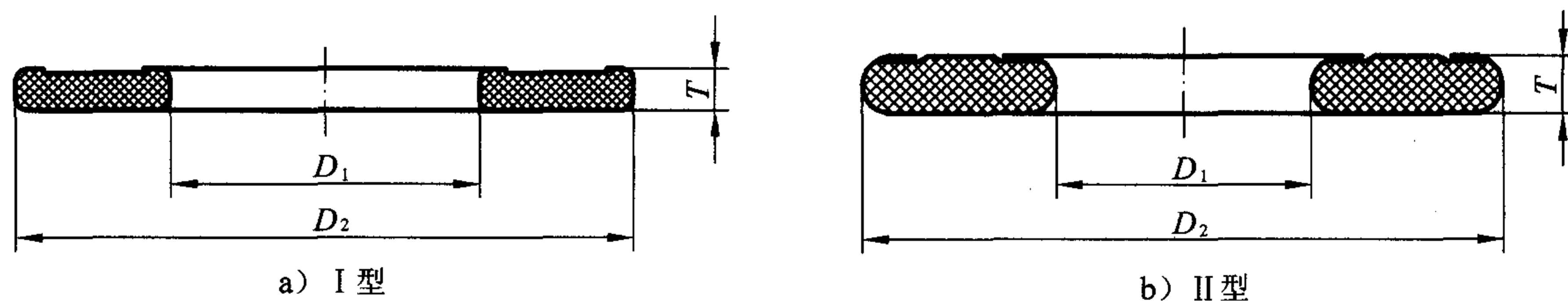
图 4.0.1 垫片的型式
